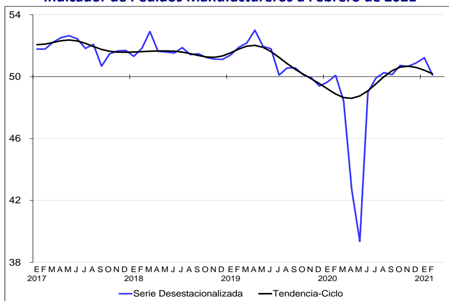
Serie Desestacionalizada y de Tendencia-Ciclo del Indicador de Pedidos Manufactureros a Febrero de 2021
